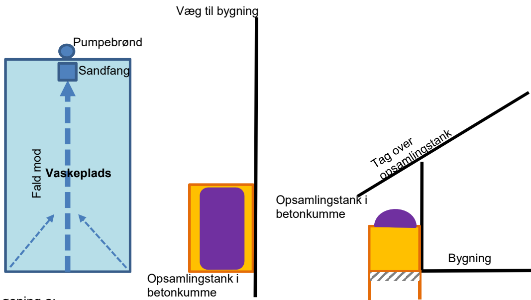
Løsning a: Plantegning - anlæg set ovenfra
