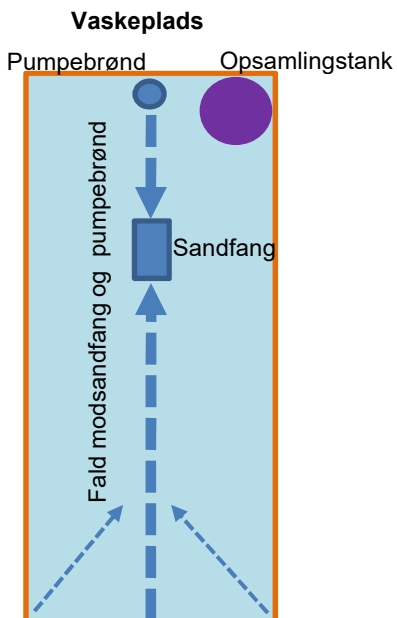
Løsning b: Plantegning - anlæg set ovenfra
